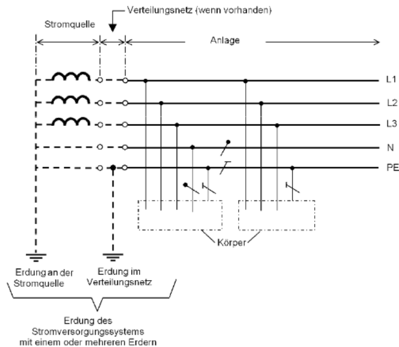
Bild 1: TN-S-System: Neutralleiter und Schutzleiter werden getrennt verlegt. (Quelle: DIN-VDE0100-100:2009-06)
